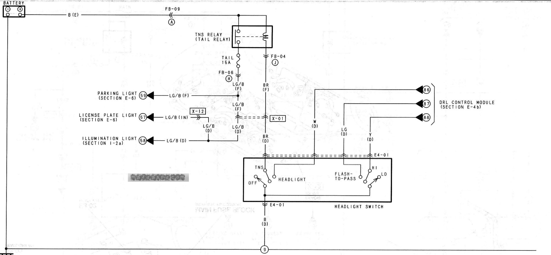
E4-01 HEADLIGHT SWITCH (D)
