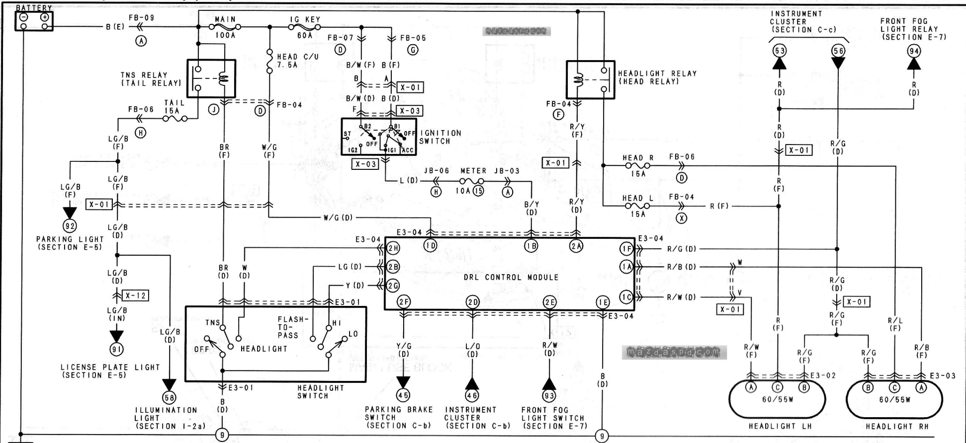
E3-01 HEADLIGHT SWITCH (D)
