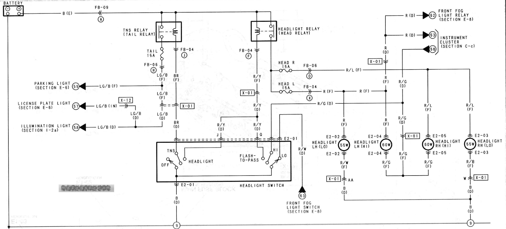
E2-01 HEADLIGHT SWITCH (D)
